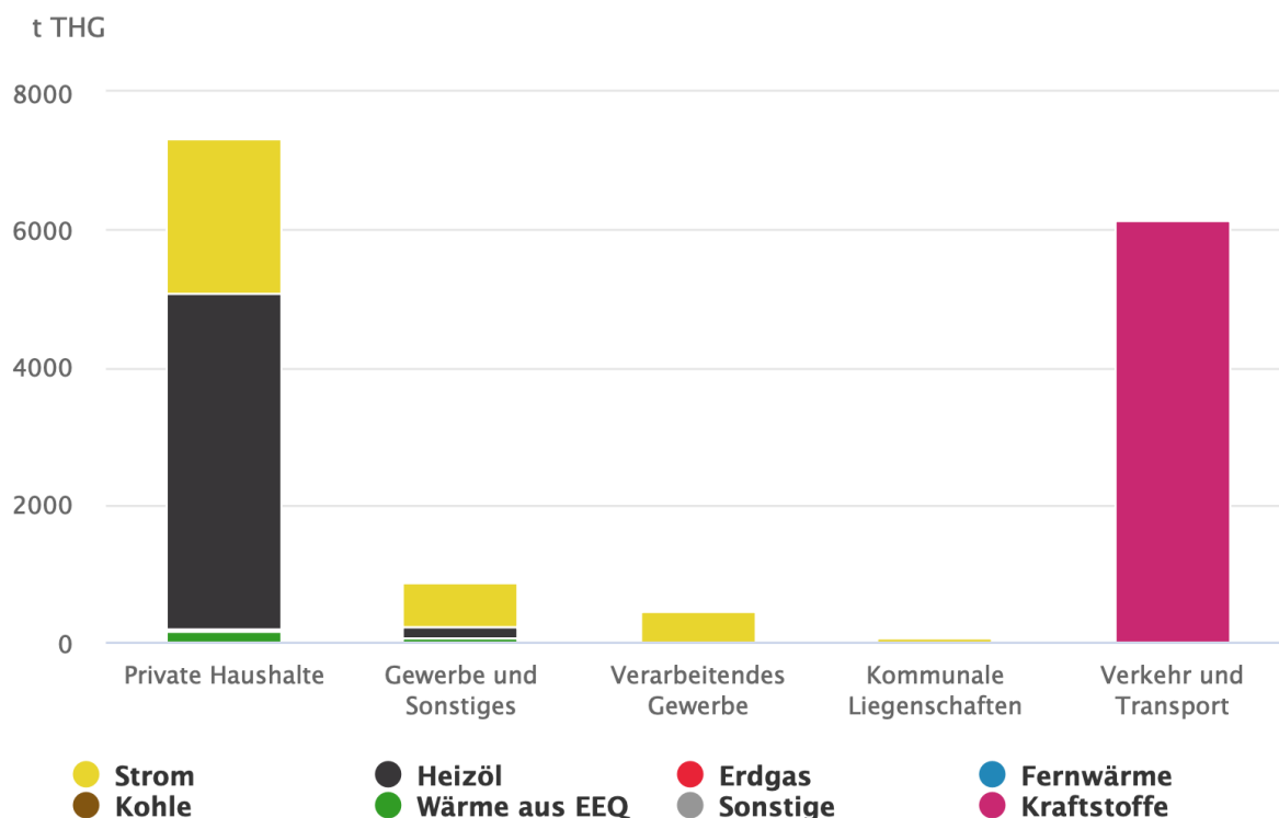
Abbildung 3-2: Ergebnis der THG-Bilanz für Heiligkreuzsteinach in t THG.
