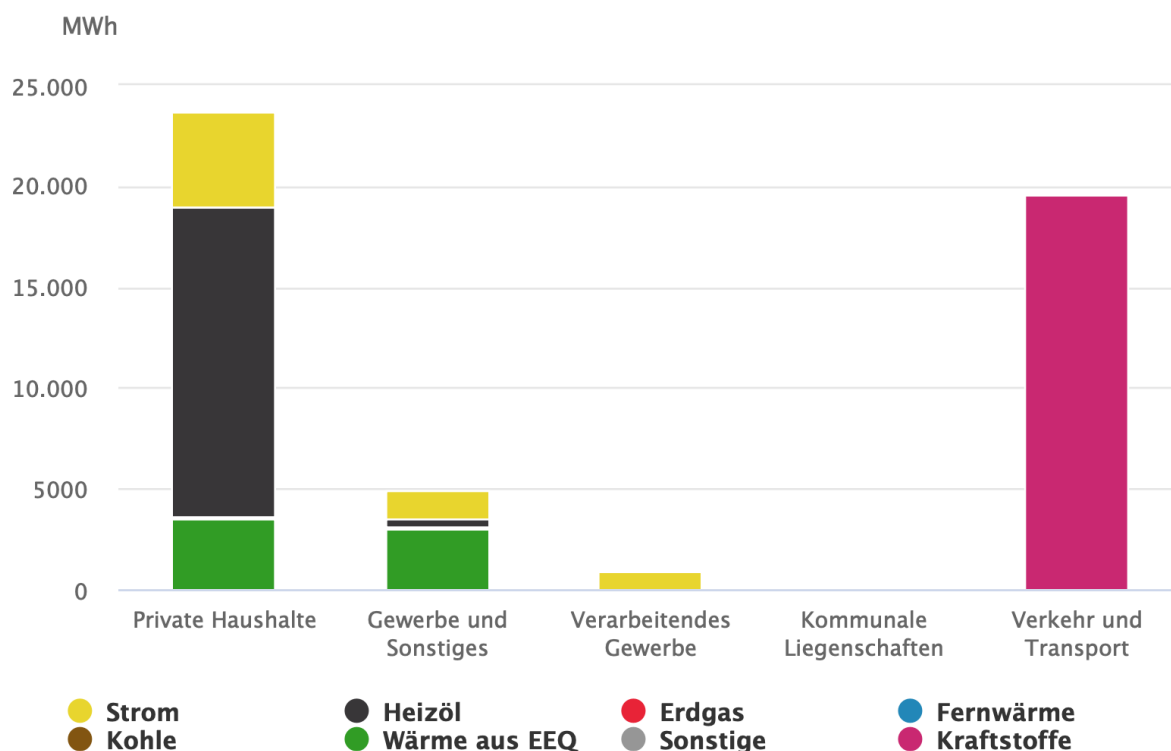
Abbildung 3-1: Ergebnis der Endenergie-Bilanz für Heiligkreuzsteinach in MWh
