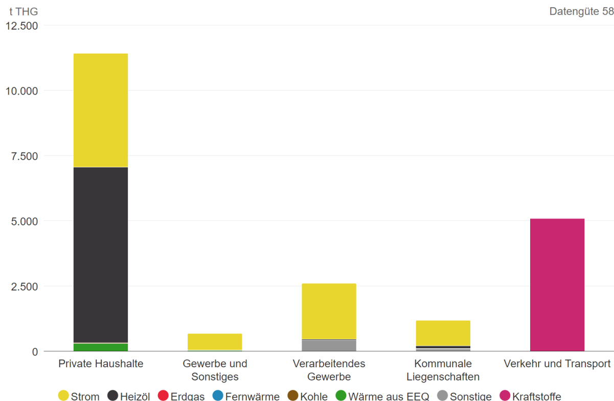
Abbildung 3-2: Ergebnis der THG-Bilanz für Schönau in t THG.
