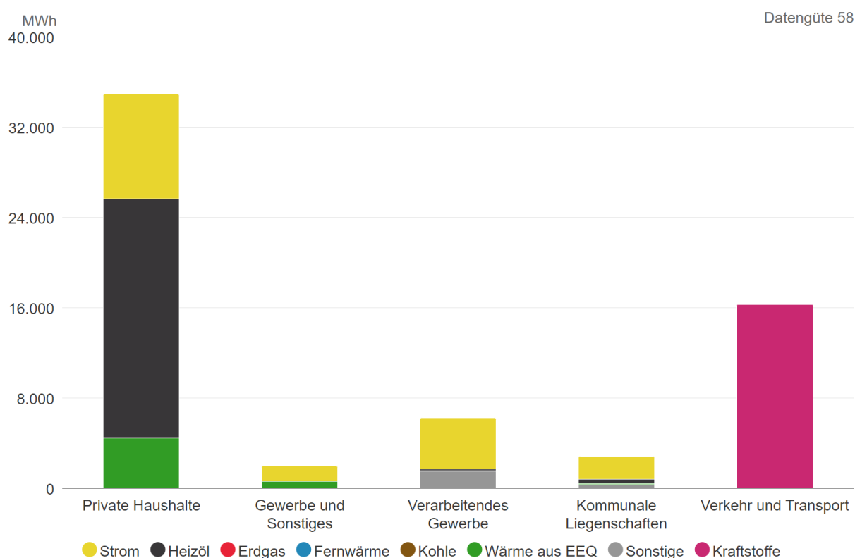
Abbildung 3-1: Ergebnis der Endenergie-Bilanz für Schönau in MWh
